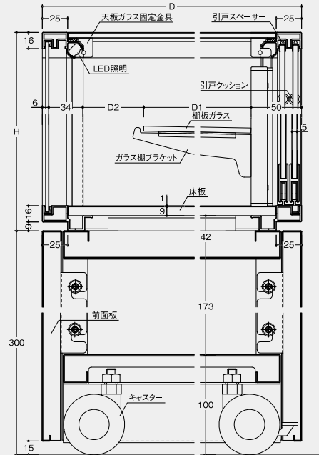
●C-C' 断面図
